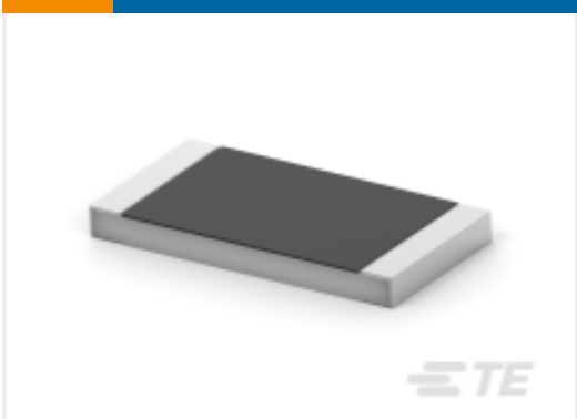
TE 产品编号1622820-3 SMD 功率电阻器：1 瓦特，3520 系列
