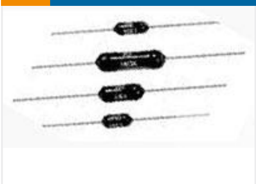
TE 产品编号1-1879623-3 H4 250R 0.1% 25PPM
