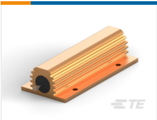
TE 产品编号1630027-1 功率电阻器：铝壳体，HSC
