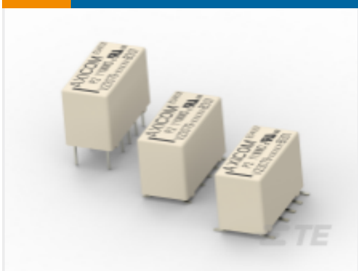
TE 产品编号2-1393788-0 AXICOM P2 标准
