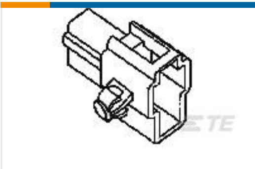
TE 产品编号172383-1 FF 250 REC HSG 2P NYLON NAT P/M
