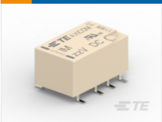
TE 产品编号1462043-3 信号继电器：2 form A，2 NO 端子
