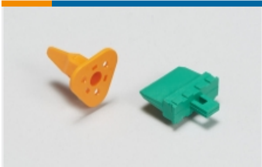
汽车接头(3)
