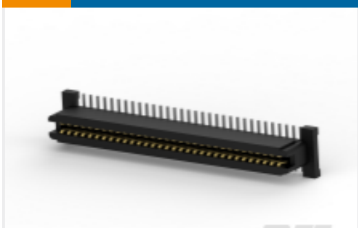
TE 产品编号120521-1 自由高度插座连接器：板对板，垂直，64，1mm
