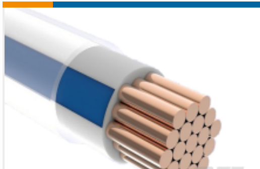
TE 产品编号F726403001 ACW0219-0.50-34(NS)
