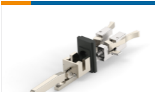
TE 产品编号2-528041-4 DIE SET, HVA 280 - 3PM HEX 9.3
