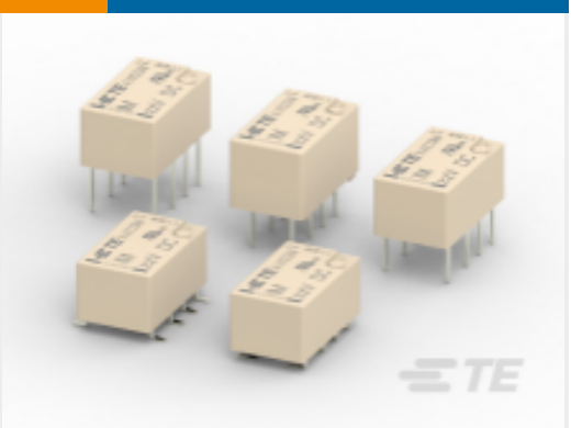
TE 产品编号4-1462037-0 标准信号继电器 2 Form C，2 CO 端子
