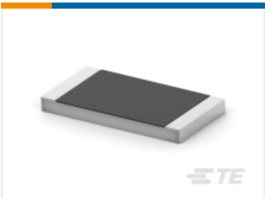
TE 产品编号2-1622820-7 SMD 功率电阻器：1 瓦特，3520 系列
