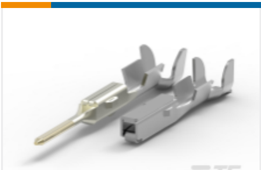
TE 产品编号1717172-1 MULTILOCK，母端和公端
