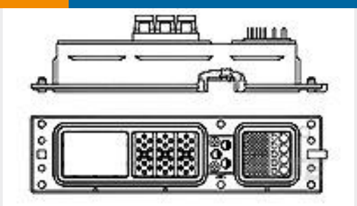
TE 产品编号1883150-2 A600 SZ 2 RCPT F36/blk/59
