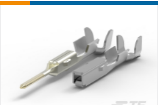
TE 产品编号1897724-1 MULTILOCK , 母端和公端
