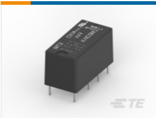
TE 产品编号1462000-7 AXICOM MT2 高灵敏型
