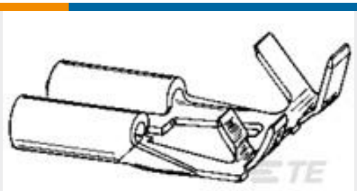
TE 产品编号179967-2 MULTILOCK，母端和公端
