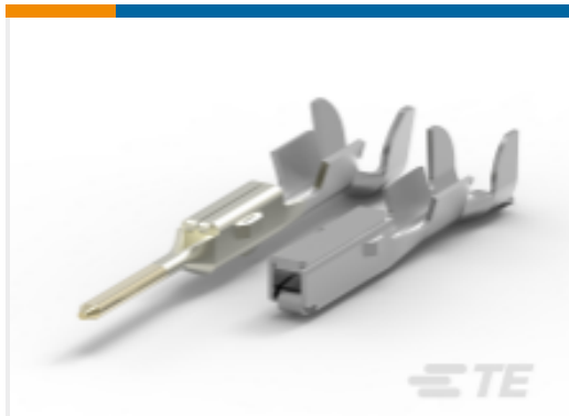
TE 产品编号1-368088-1 MULTILOCK，母端和公端
