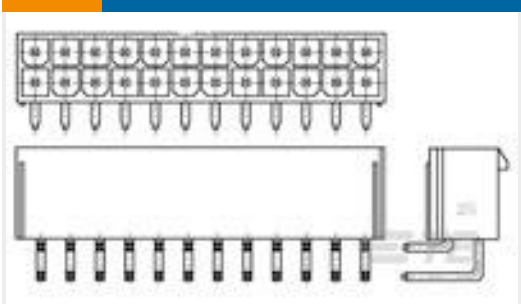
TE 产品编号1586863-4 4P VAL-U-LOK R/A HDR GW
