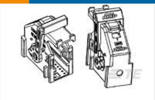
TE 产品编号174979-1 信号接头
