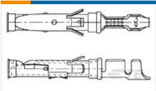
TE 产品编号163767-5 062 SOC.ASS.TYPE 3+
