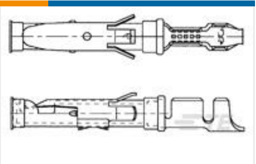
TE 产品编号163767-4 062 SOC.ASS.TYPE 3+
