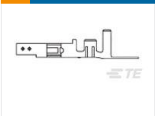
TE 产品编号1586315-4 VAL-U-LOK SKT PHBZ AU 24-18 LP
