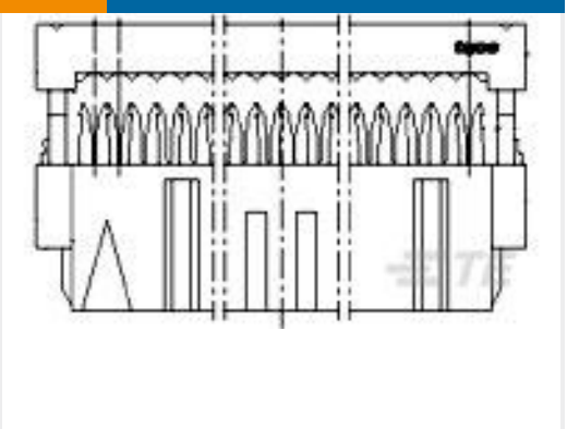
TE 产品编号2-215882-0 20 WAY GREY MK II RECP
