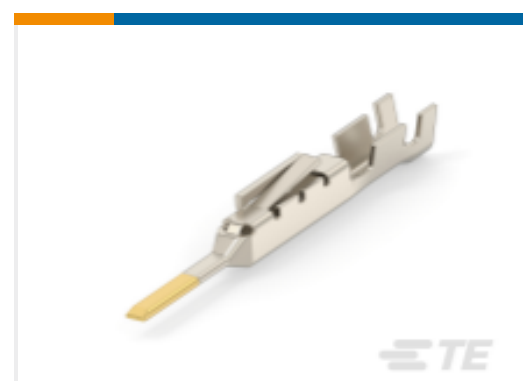
TE 产品编号1318109-1 Dynamic 2000 端子
