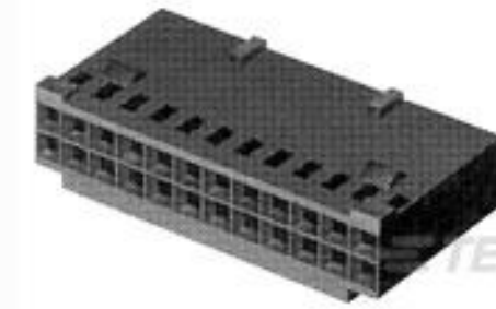
TE 产品编号 1-87631-5 20 MODIV HSG COMP DR .100 POL
