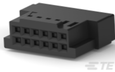
TE 产品编号487769-7 2.54mm FFC 连接器母端外壳
