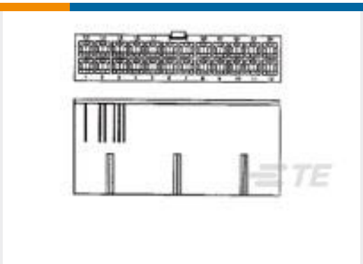
TE 产品编号1586017-4 4P FH PLUG VAL-U-LOK V0
