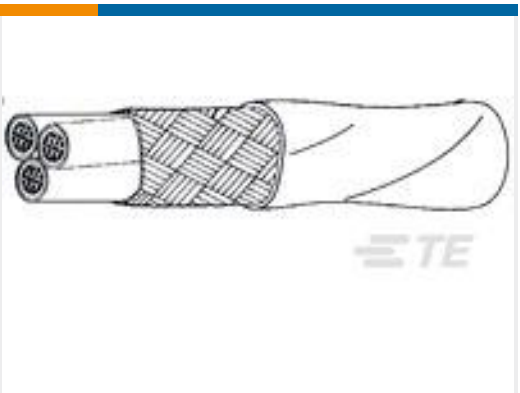
TE 产品编号382308-004 44A1131-16-0/2/9-9
