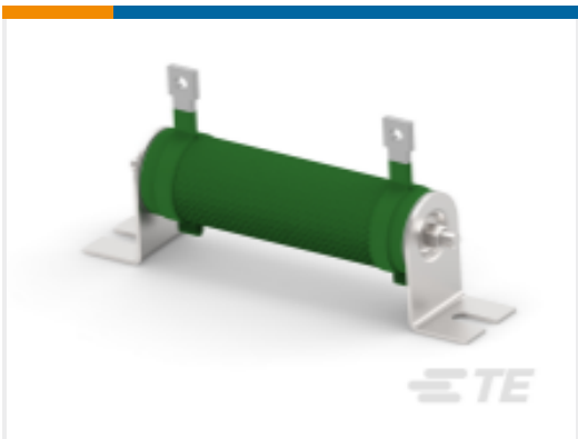
TE 产品编号1879452-1 线绕电阻器：矿物，2.5 Kw
