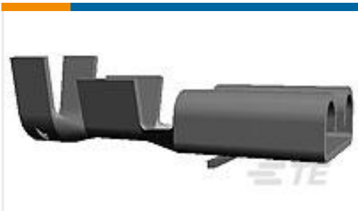
TE 产品编号160917-2 FF 250 REC 1-2.5MM2 TPBR
