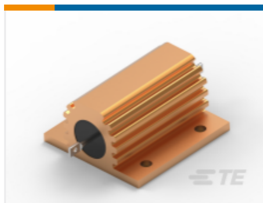
TE 产品编号3-1630024-7 功率电阻器：铝壳体，HSA
