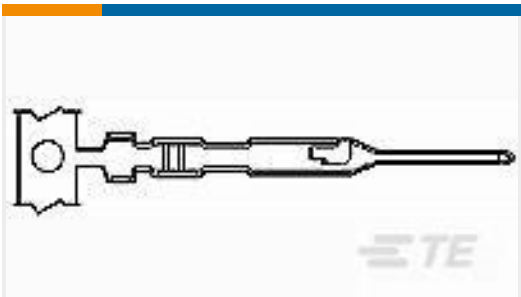
TE 产品编号104505-2 MTE PIN 22-26 AWG PLTD
