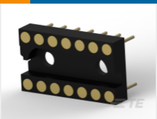
TE 产品编号1-1437531-7 DIP 插座：标准，自动车床，封闭式，镀金
