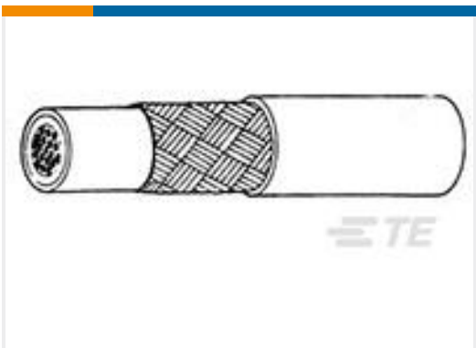
TE 产品编号556070-000 55A1113-20-9-9
