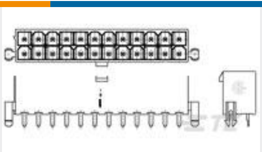
TE 产品编号2-1586039-2 22P VAL-U-LOK VRT HDR W/P V2
