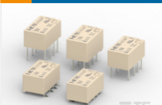
TE 产品编号1-1462039-9 标准信号继电器 2 Form C，2 CO 端子
