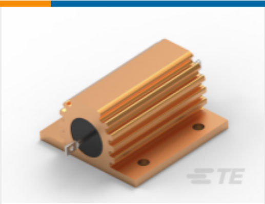
TE 产品编号1-1625984-1 功率电阻器：铝壳体，HSA
