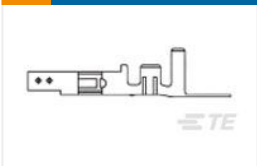
TE 产品编号1586317-3 VAL-U-LOK SKT PHBZ SN 26-22 LP
