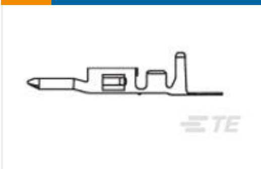
TE 产品编号1586314-3 VAL-U-LOK PIN PHBZ SN 24-18 LP
