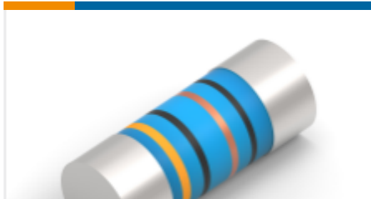
TE 产品编号1-2176316-6 MELF SMA_A 1K8 0.1% 15PPM 0207 1W
