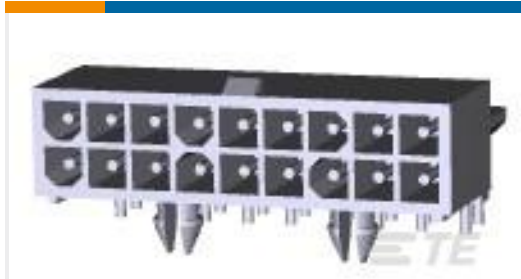
TE 产品编号1-794105-0 18P MINI UMNL R/A HDR ASSY SN
