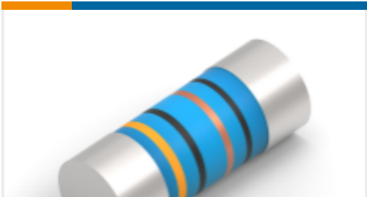
TE 产品编号1-2176316-4 MELF SMA_A 1K2 0.1% 15PPM 0207 1W
