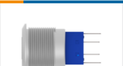
TE 产品编号1-2316542-3 AV19 DPM 3A SPOT LOGO R&G 12V
