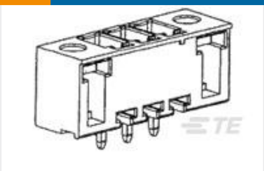
TE 产品编号1-284516-2 12P TERMIBLOK HDR DIR C VITI
