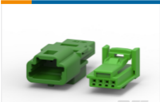
TE 产品编号1473672-1 TH/025 连接器系统, 壳体
