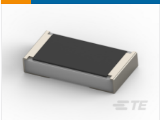
TE 产品编号1-2176230-2 SMD 功率电阻器：3 瓦特，1% Tol
