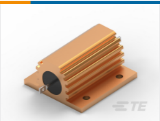
TE 产品编号5-1630186-7 功率电阻器：铝壳体，HSA
