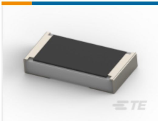
TE 产品编号1-2176230-0 SMD 功率电阻器：3 瓦特，1% Tol
