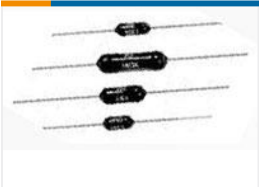
TE 产品编号4-1879619-9 H8 1K0 1% 25PPM
