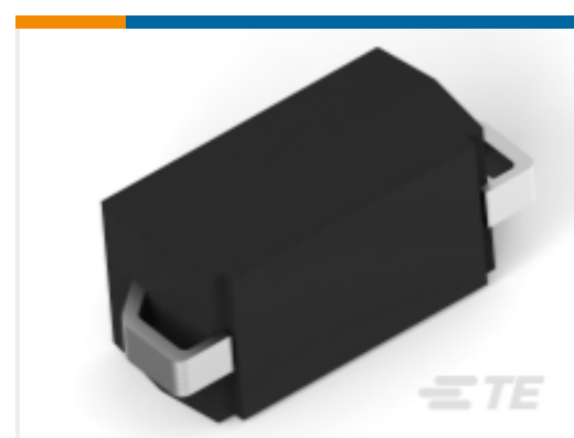
TE 产品编号1-2176324-9 SMV 3W 3M3 5%
