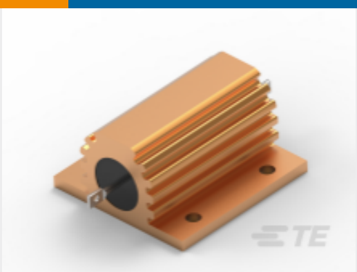
TE 产品编号1625984-7 功率电阻器：铝壳体，HSA
