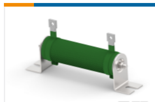
TE 产品编号1879453-4 线绕电阻器：矿物，2.5 Kw
