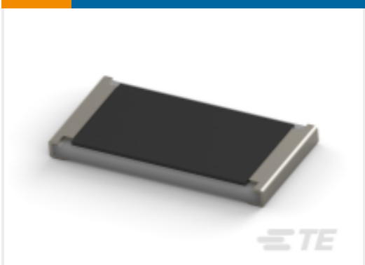
TE 产品编号1-2176070-7 SMD 功率电阻器：2 瓦特，3521 系列
