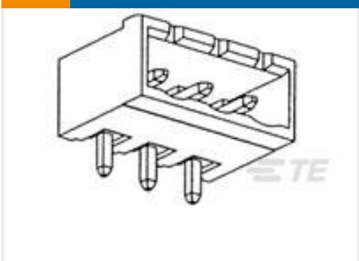
TE 产品编号1546109-2 EUROSTYLE TB,HEADER,GREY,2 POS
