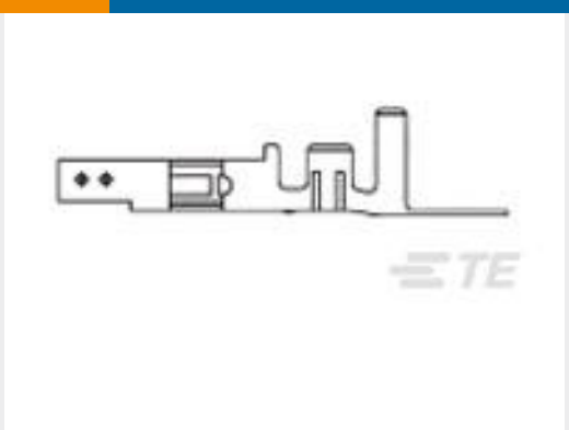
TE 产品编号1586317-1 VAL-U-LOK SKT BR SN 26-22 LP
