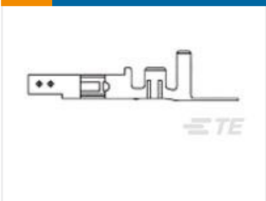
TE 产品编号794958-1 VAL-U-LOK SKT BR SN 22-26AWG
