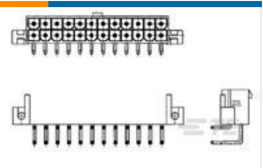
TE 产品编号1586043-8 8P VAL-U-LOK R/A HDR SCR MT V2
