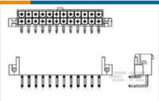
TE 产品编号2-1586043-4 24P VAL-U-LOK R/A HDR SCRMT V2
